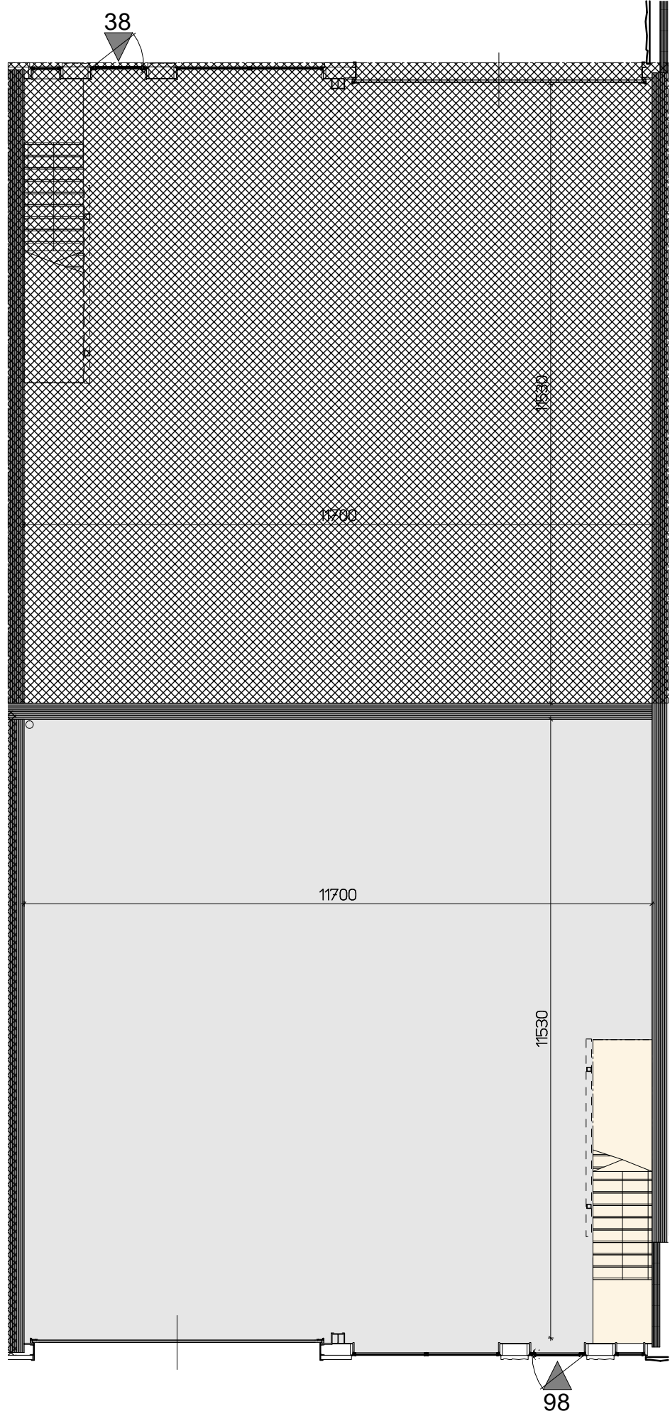
Begane grond
